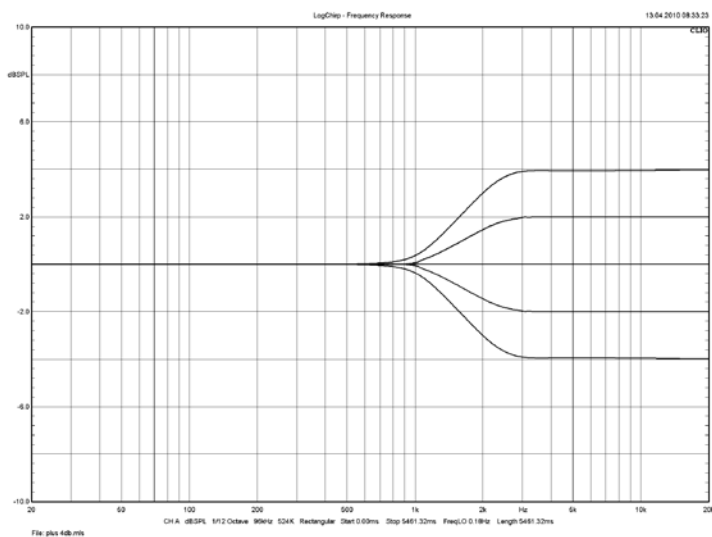
fig. 8: Tweeter Level
