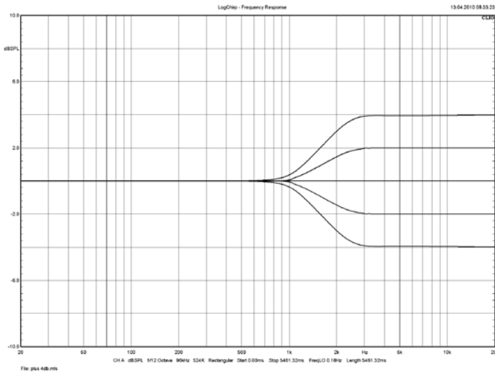
Abb. 8: Hochtonpegel
