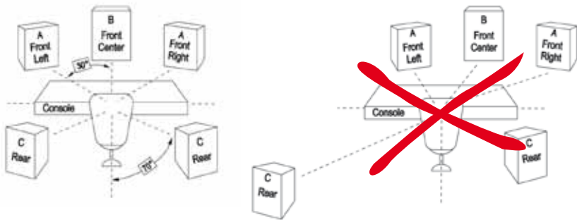
Abbildung 7: Surround-Anordnung
