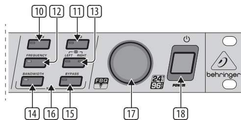
Rys. 3.3: Elementy obsługi po prawej stronie FBQ2496
