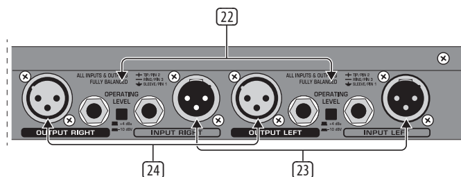
Rys. 3.6: Gniazda na panelu tylnym procesora FBQ2496
