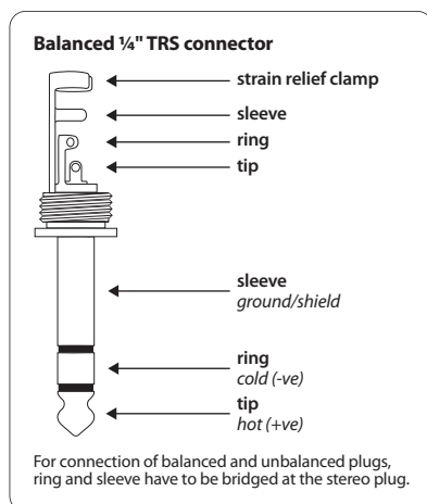
Rys. 8.1: Stereofoniczny wtyk jack 6,3 mm
