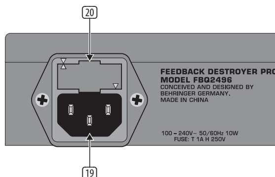
Rys. 3.4: Gniazdo zasilania, bezpiecznik i numer seryjny
