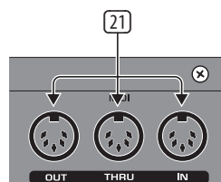
Rys. 3.5: Gniazda MIDI procesora FBQ2496
